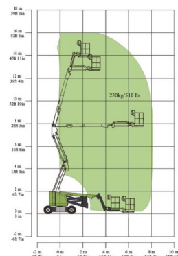
ZA14JE(-Li)作業範囲図
