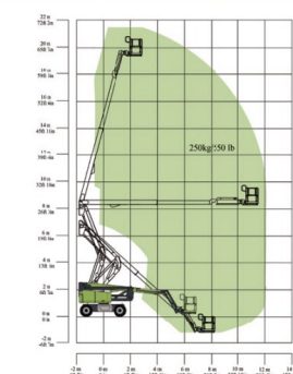
ZA20JE作業範囲図
