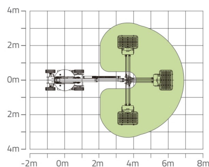
ZA10RJE作業範囲図
